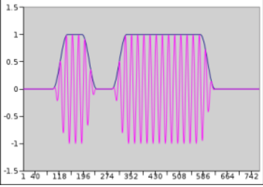
Figure 2.115 Dash/Dot = 3.0, Edge = 6 msec
